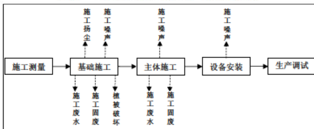
图4-2 项目开关站施工期工艺流程及产污环节示意图
