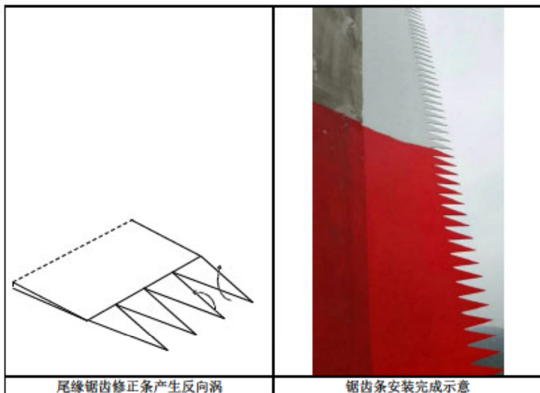
图 4-4 风机尾缘锯齿条示意图
